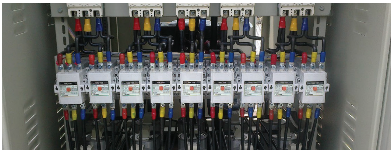
TỦ TỤ BÙ CÔNG SUẤT PHẢN KHÁNG
